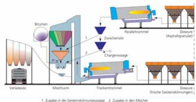
Mischanlagenschema mit Paralleltrommel (Quelle: Deutscher Asphaltverband)
