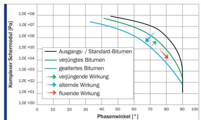
Bitumenalterung und -verjüngung im Black-Diagramm
